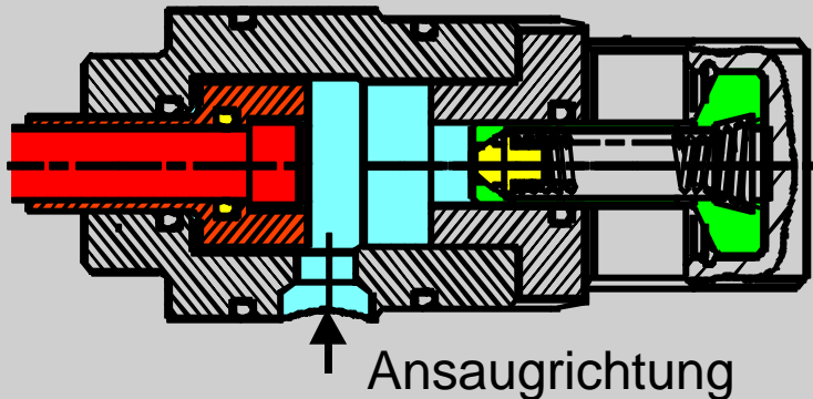
2. Komprimierungsphase Beginn
