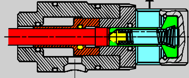
4. Förderphase
