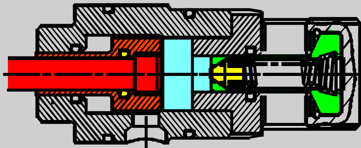
2. Komprimierungsphase Beginn
